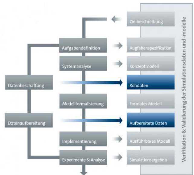
V&V Vorgehensmodell
