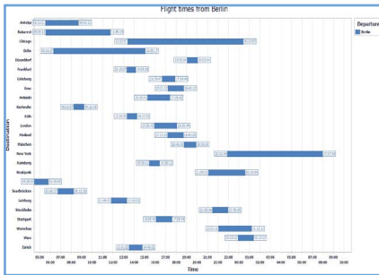
SimGantt
